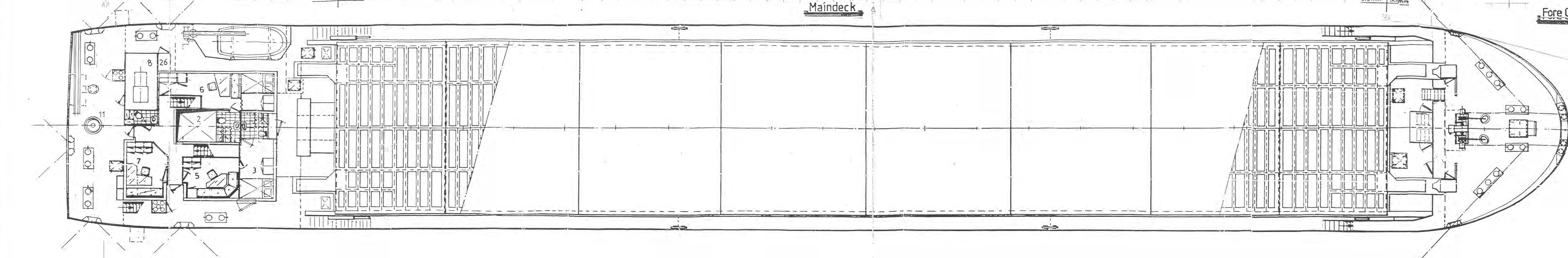
Tweendeck
